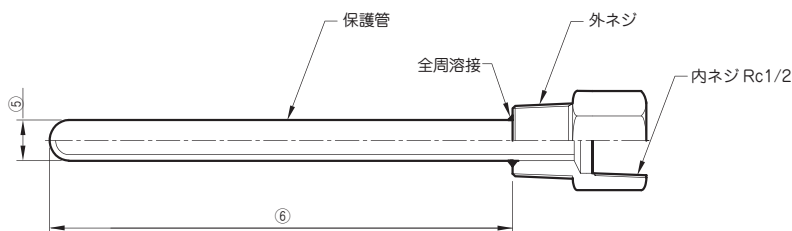
外径図
